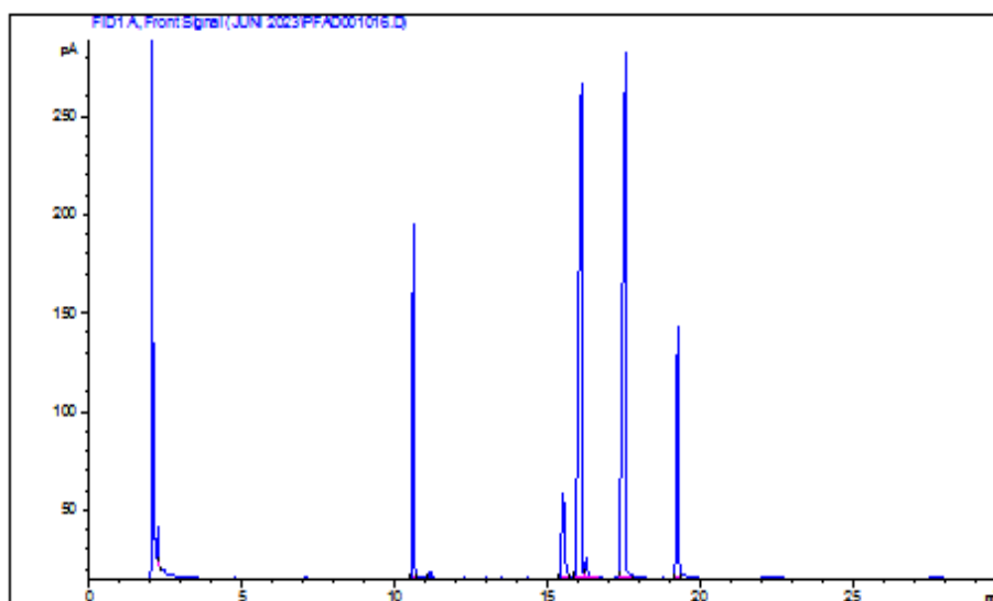
Gambar 2. Kromatografi hasil uji GC-FID
