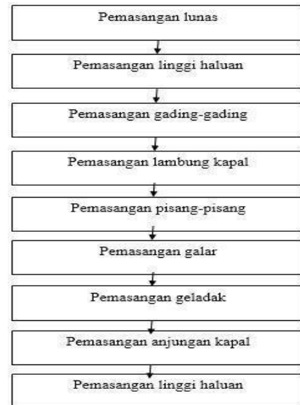
Gambar 2. Proses pembangunan kapal kayu.
