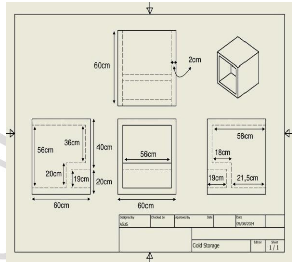
Lampiran 2. Desain cold storage gambar teknik.
