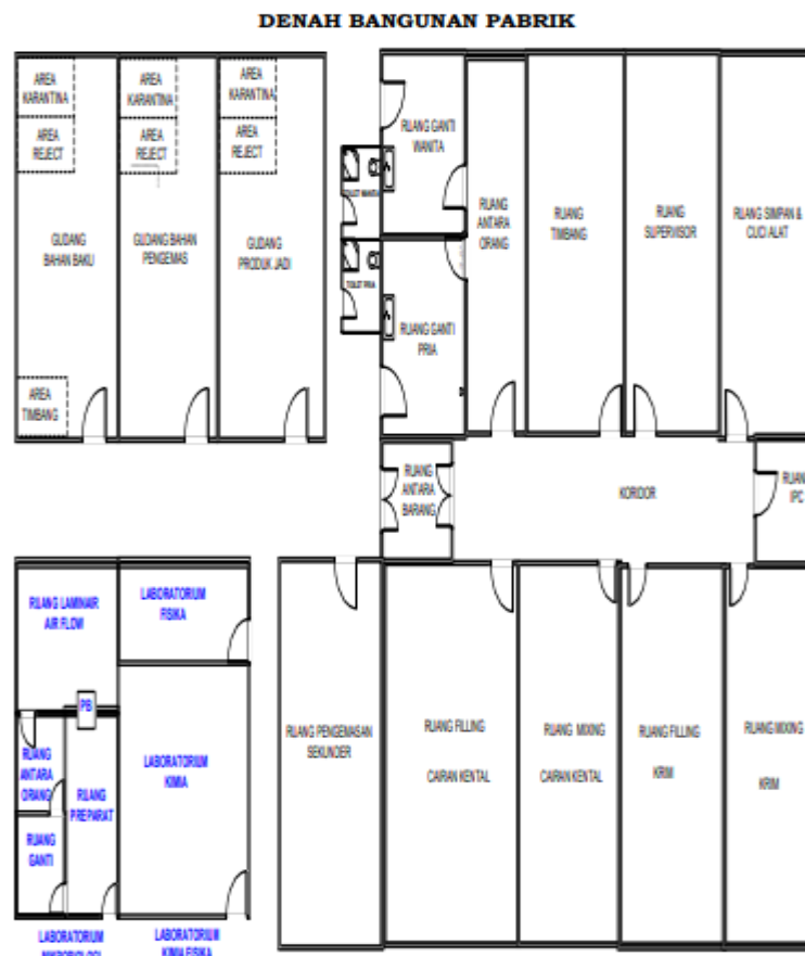
Gambar 2.2.4.2 Denah Bangunan Pabrik
