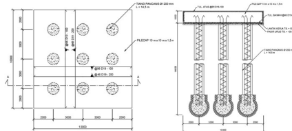
Gambar 12. Dimensi Pilecap Jembatan
