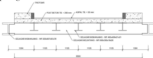
Gambar 4. Tampak Potongan Melintang Gelagar Memanjang
