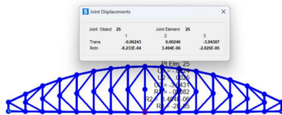
Gambar 7. Lendutan Akibat BGT
