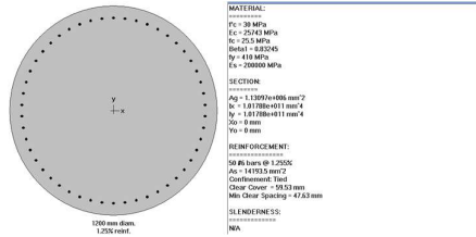
Gambar 13. Dimensi dan Material Tiang Pancang SpColumn
