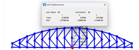
Gambar 9. Lendutan Akibat Beban Truk
