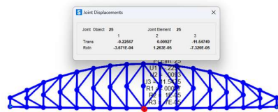
Gambar 8. Lendutan Akibat Lajur D
