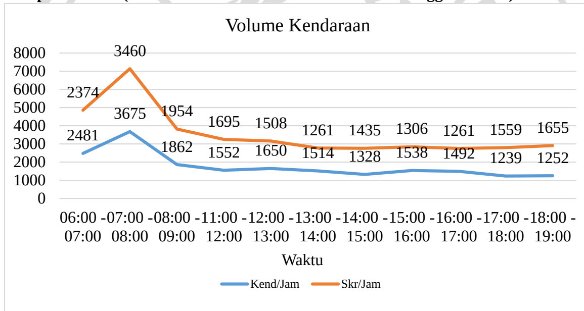
Lampiran Ke 26 (Grafik Volume Kendaraan Hari Senin Minggu Ke Dua)
