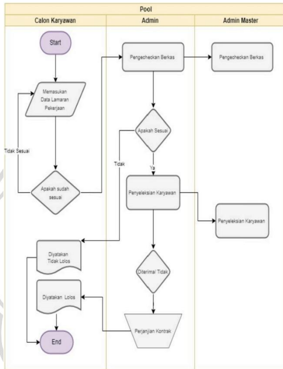
Gambar 2. 2 Flowchart sistem penerimaan pekerja berbasis web
