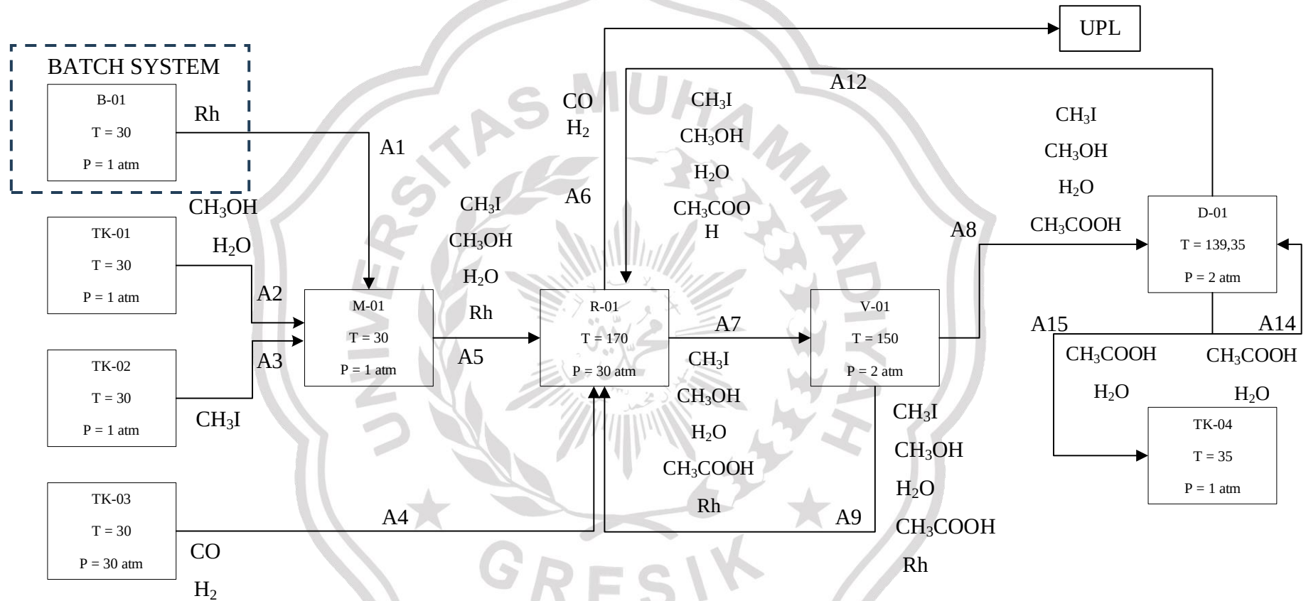
Gambar 4. 1 Diagram Alir Kualitatif
