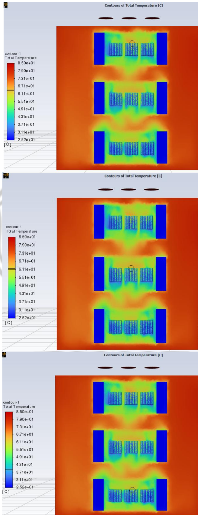
Lampiran 1. Kontur total temperatur potongan sumbu ZX oven 4 exhaust layer 2.
