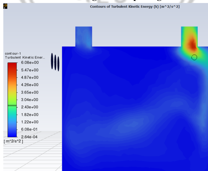
Lampiran 8. Kontur turbulen energi kinetik potongan sumbu YZ oven 4 exhaust.
