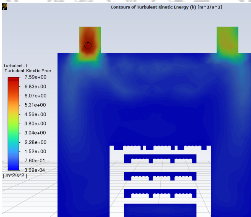
Lampiran 16. Kontur turbulen energi kinetik potongan sumbu ZX oven 2 exhaust.
