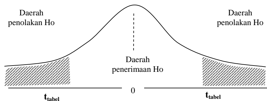
Gambar 3.2 Kurva Uji t
