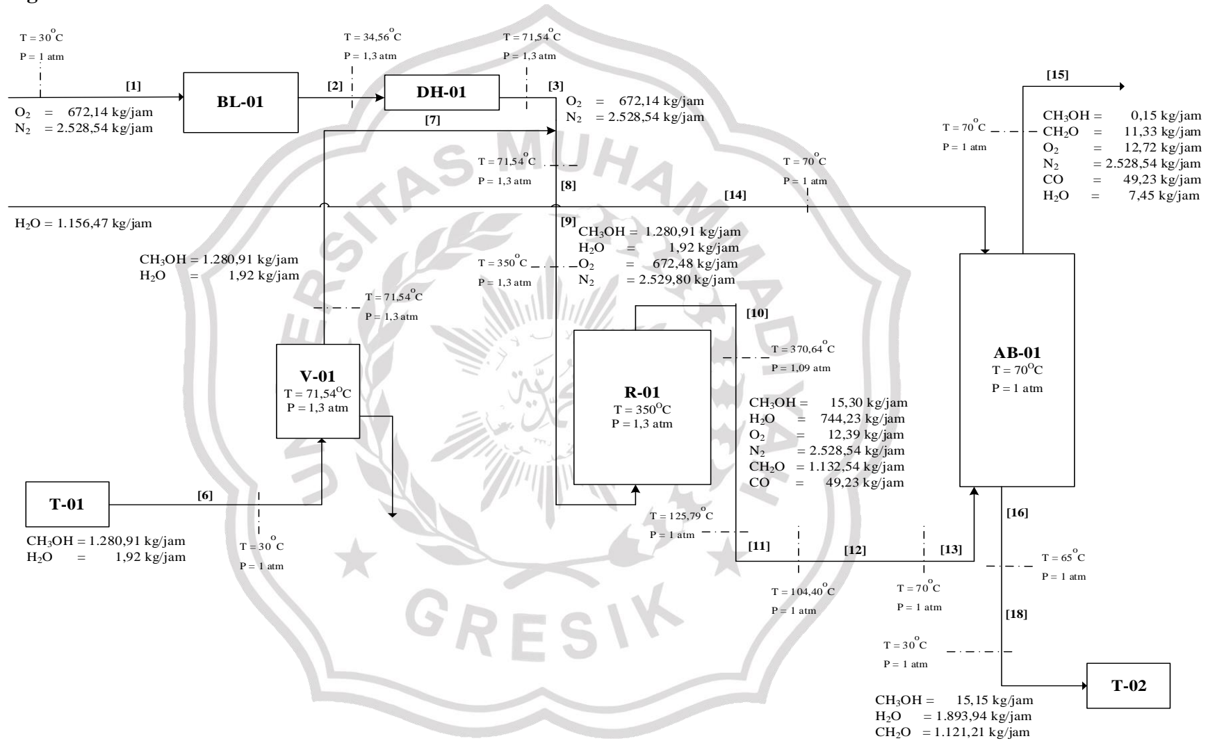
Gambar 4. 2. Diagram Blok Kuantitatif
