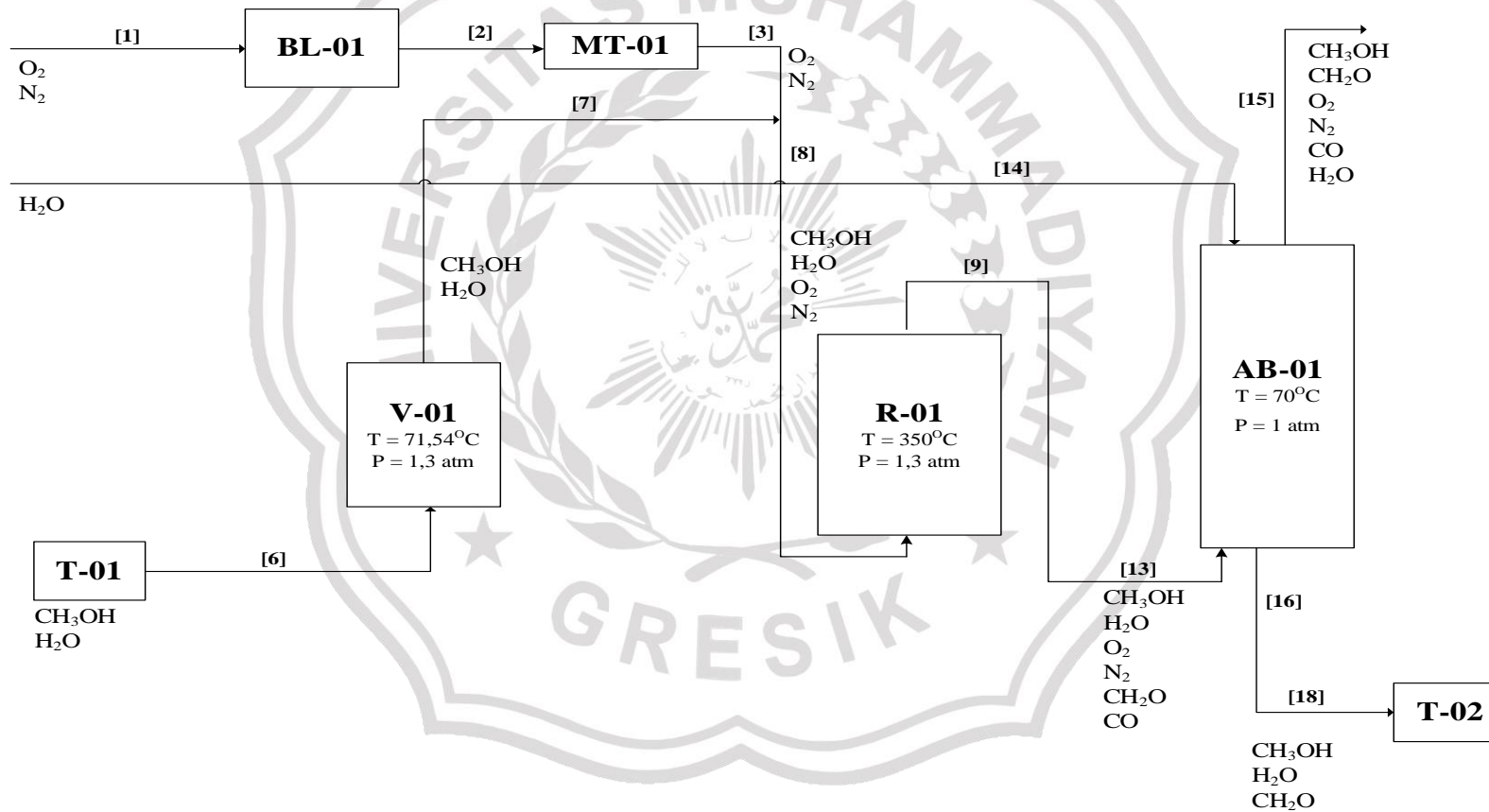
Gambar 4. 1. Diagram Blok Kualitatif
