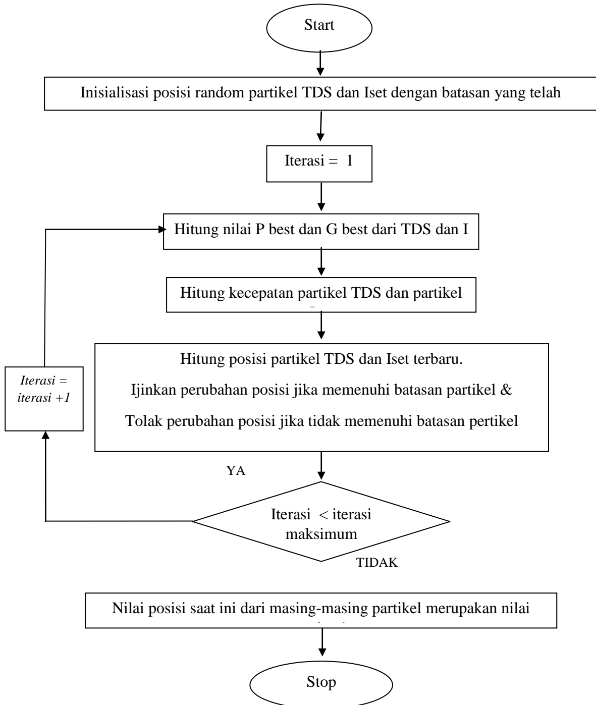
Gambar 3.2 Flow chart koordinasi rele dengan PSO
